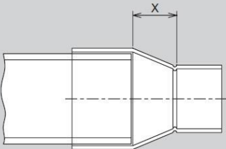
●異径ソケット
