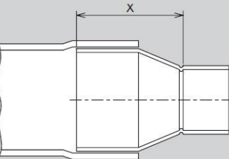
●レデューサ
